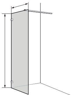
Stacionari dušo sienelė 2000x700x8 mm 2000x800x8 mm 2000x900x8 mm
